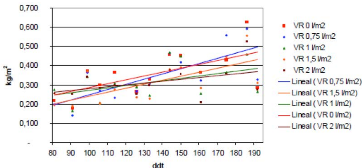
Figura 4. Líneas de tendencia la producción de tomate en el tiempo en el invernadero comercial de San Isidro de Níjar (Almería).(*)ddt: días después del transplante, VR 0 l/m 2 retransqueo + solarización, VR 0,75 l/m 2 retransqueo + 0,75 l/m 2 vinazas de remolacha + solarización, VR 1 l/m 2 retransqueo + 1 l/m 2 vinazas de remolacha + solarización, VR 1,5 l/m 2 retransqueo + 1,5 l/m 2 vinazas de remolacha + solarización, VR 2 l/m 2 retransqueo + 2 l/m 2 vinazas de remolacha + solarización).
