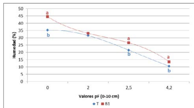
Figura 3. Contenido de humedad a diferentes presiones de succión (pF) para el perfil de suelo 0-10 cm. Valores medios ( n=3 ), de un mismo pF, con la misma letra, o sin letra, no difieren significativamente entre sí según prueba LSD de Fisher ( p<0,05 ). T: testigo. B1: biosolarización de primer año.
